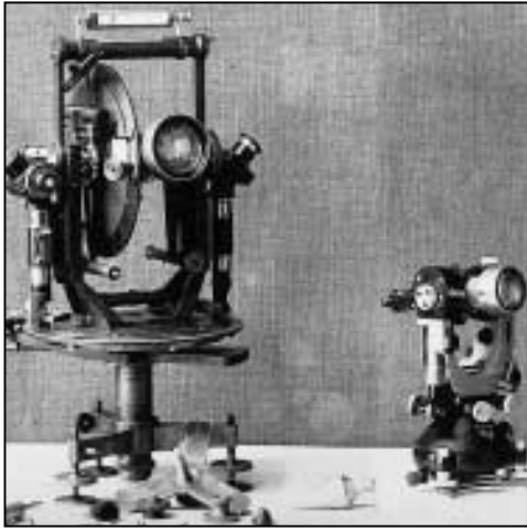
Ein Vergleich: Der kleine Universalthedolit Wild T2 löste die gleichen Aufgaben wie der Triangulations-Theodolit vorheriger Bauart – und war trotz seiner Kompaktheit genauer und zuverlässiger.
